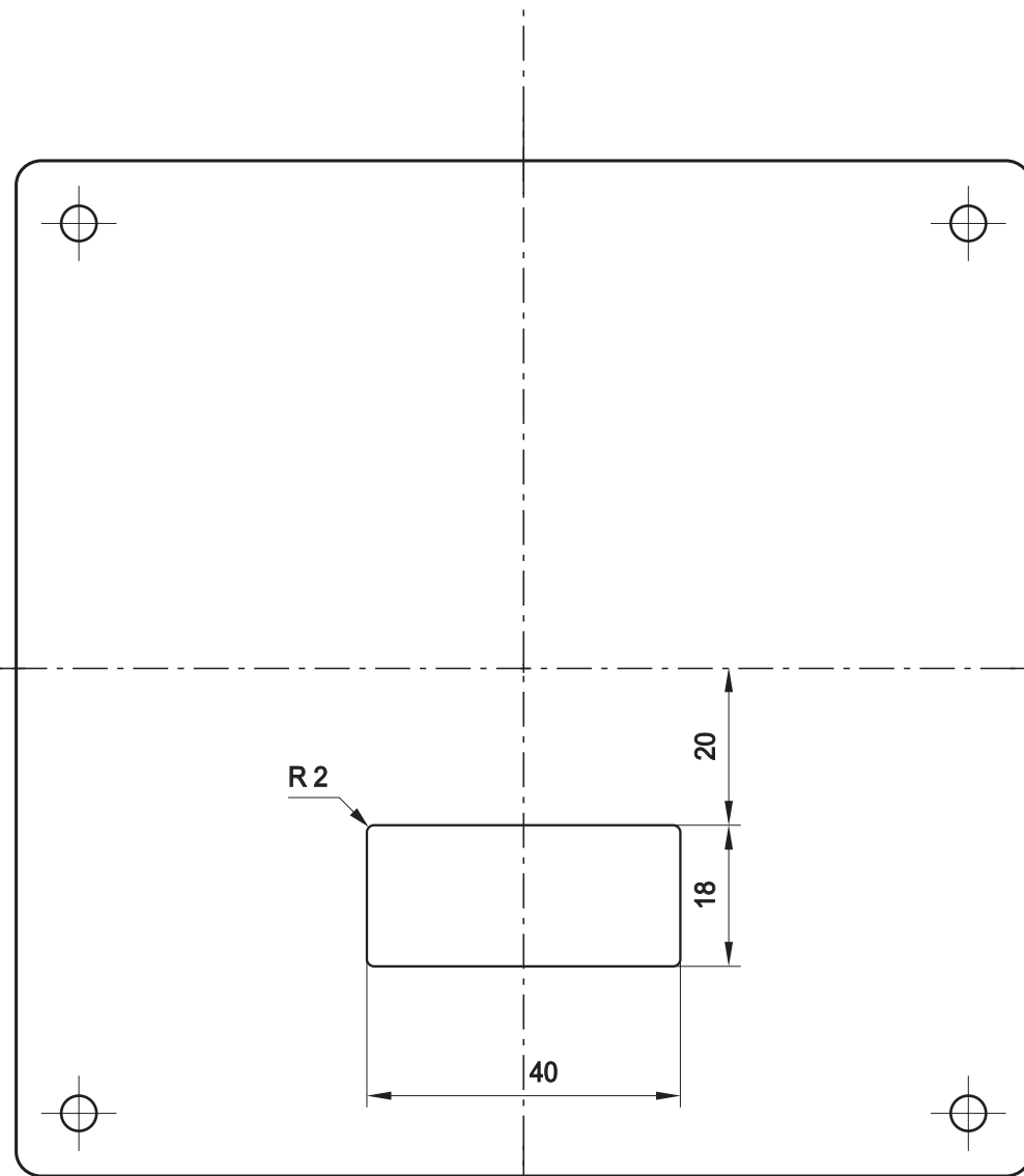
Szablon do trasowania otworów obudowy BB05
